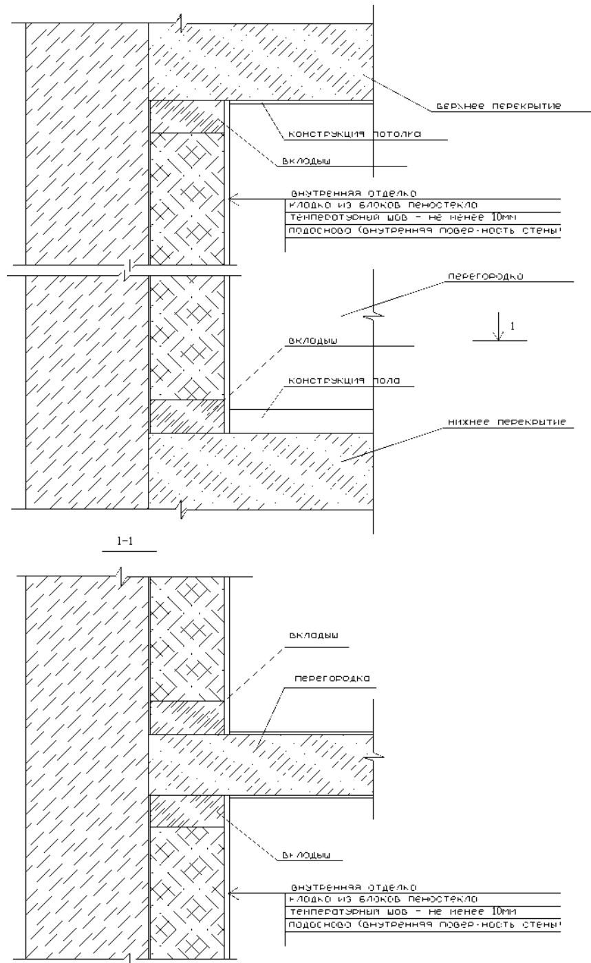
Рисунок А.6 – Внутренняя тепловая изоляция стен
