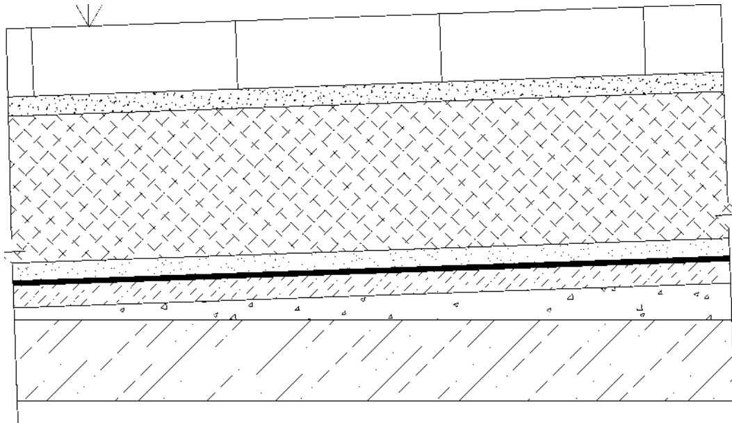
Рисунок А.21 – Тепловая изоляция в инверсионной кровле
