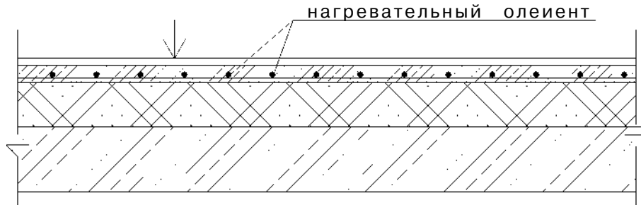
Рисунок А.7 – Тепловая изоляция пола из пенокрошки на перекрытии
