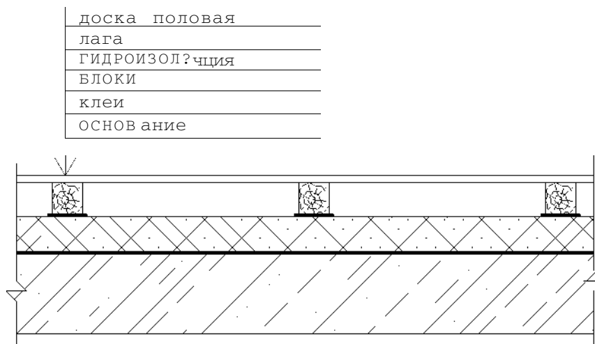
Рисунок А.12 – Тепловая изоляция дощатого пола
