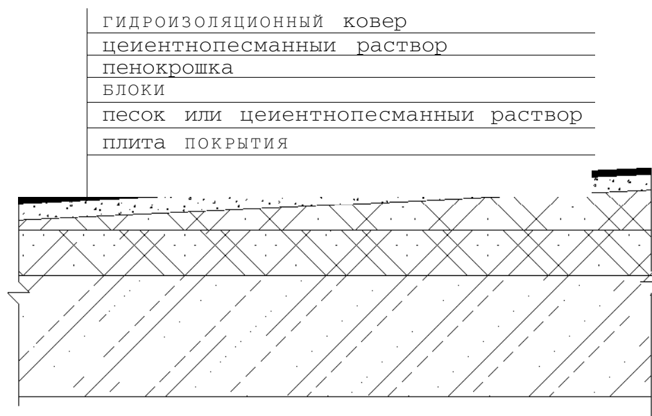
Рисунок А.19 – Тепловая изоляция совмещенной плоской кровли из блоков с разуклонкой из пенокрошки
