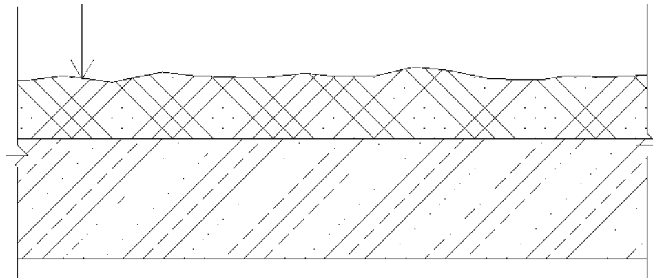
Рисунок А.25 - Тепловая изоляция не эксплуатируемого чердачного перекрытия
