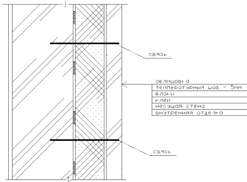
Рисунок А.1 – Тепловая изоляция трехслойной стены
