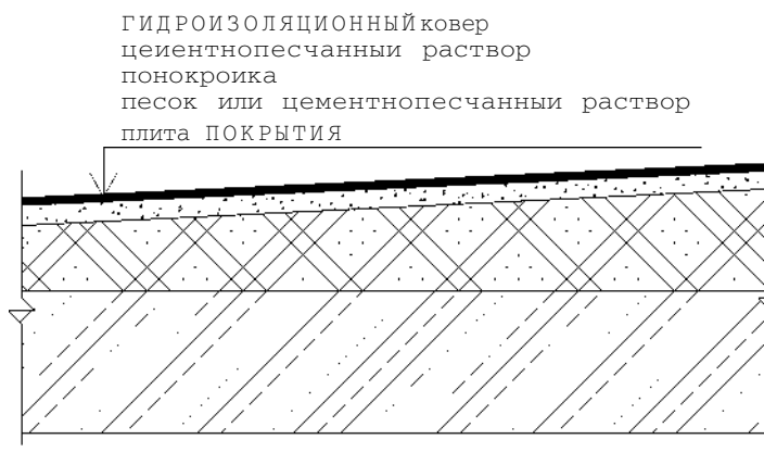
Рисунок А.16 – Тепловая изоляция совмещенной плоской кровли из пенокрошки
