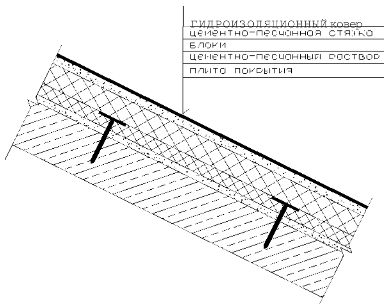
Рисунок А.18 – Тепловая изоляция совмещенной кровли с уклоном более 25%
