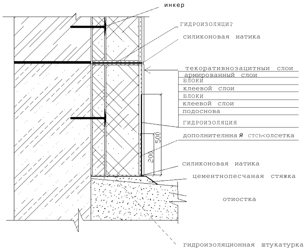
Рисунок А.26 - Тепловая изоляция цоколя выше отмостки
