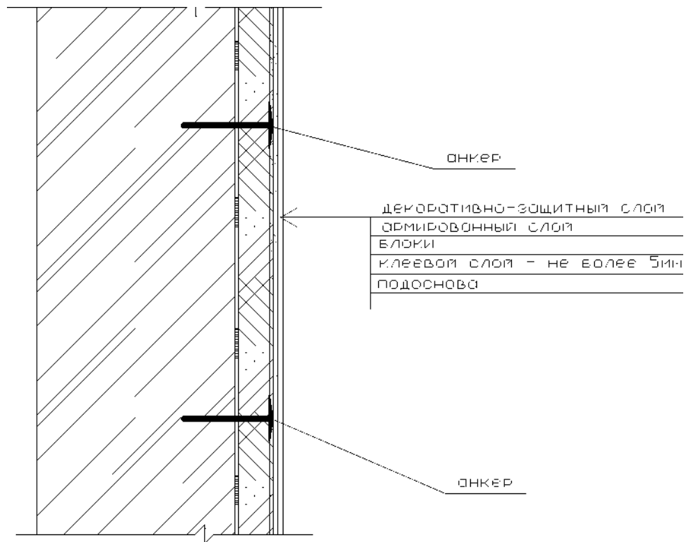
Рисунок А.3 – Легкая штукатурная система утепления стен из блоков в один слой
