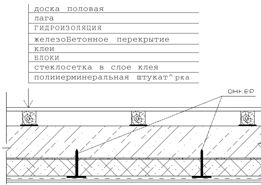
Рисунок А.14 – Наружная тепловая изоляция перекрытия с отделкой полимерминеральными материалами
