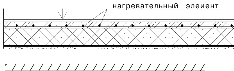
Рисунок А.8 - Тепловая изоляция пола из блоков на перекрытии
